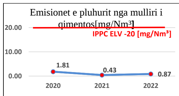
Figure 3 Emisionet e Pluhurit nga mulliri i çiment
