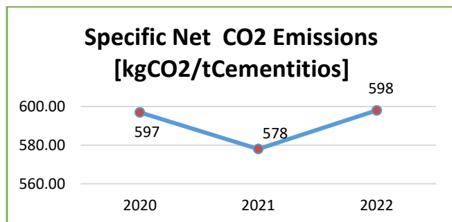
Figure 9 Emisionet specifike te CO2 per produkte te cimentos
