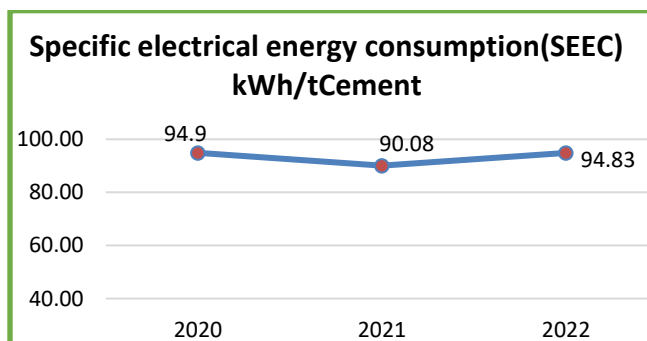
Figure 3 Hargjimi specifik i energjise elektrike per prodhim te cimentos
