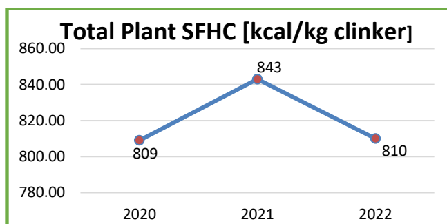
Figure 8 Hargjimi specifik i nxehtesise për prodhim të clinkerit
